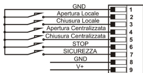
Morsetteria ingressi
