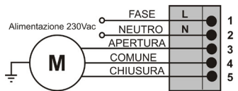
MOTORE a 230Vac Morsetteria aliment. di rete e motore
