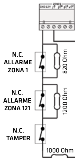
CONTATTO N.C. DI ALLARME ZONA 1, CONTATTO N.C. DI ALLARME ZONA 121 E CONTATTO N.C. DI TAMPER CON RESISTENZE DI TRIPLO BILANCIAMENTO
