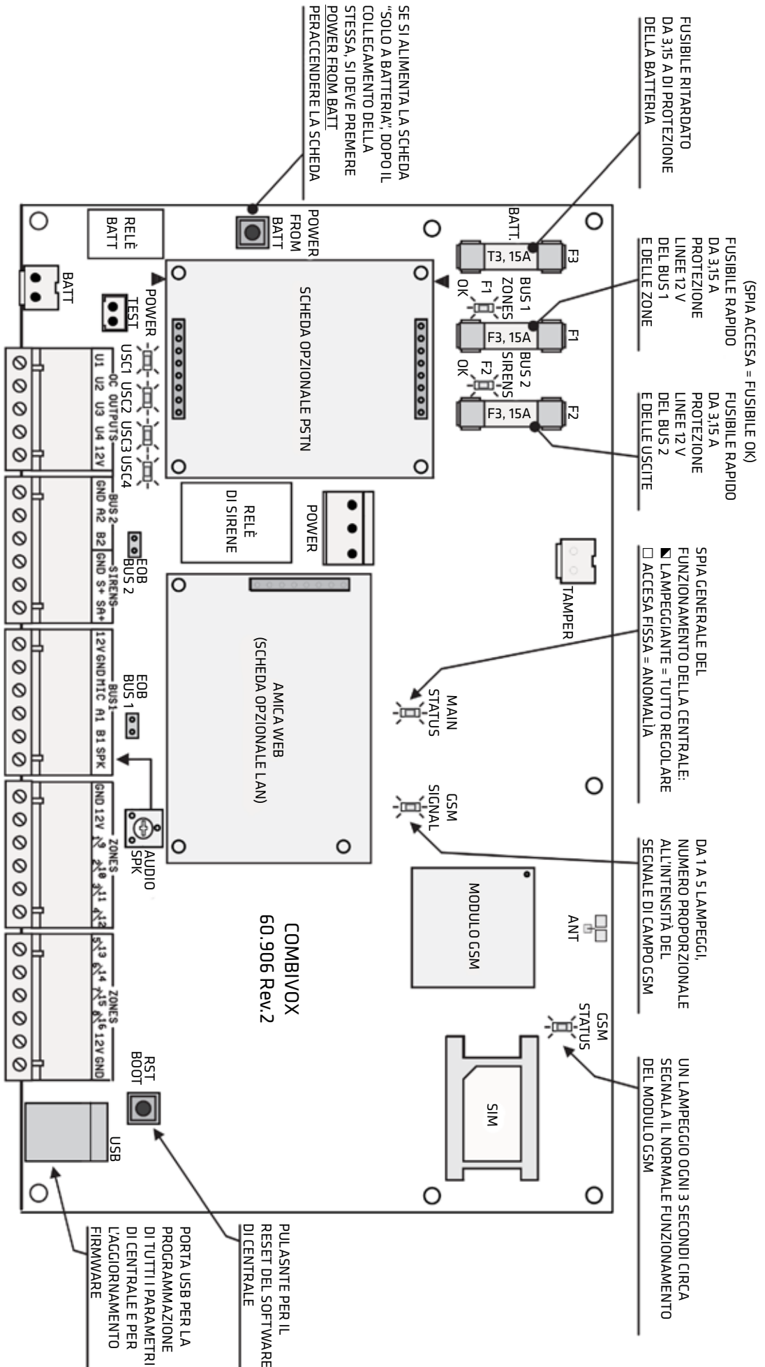
IMPORTANTE: LA CENTRALE SI ACCENDE SOLO TRAMITE L'ALIMENTATORE SWITCHING COLLEGATO ALLA RETE 220 V E RIMANE SPENTA SE SI UTILIZZA LA SOLA BATTERIA Figura 1: Schema della Amica 64 con descrizione di fusibili, spie, morsetti e pulsanti
