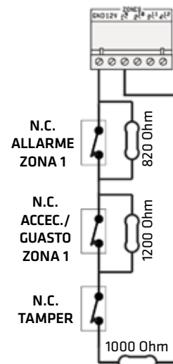
CONTATTO N.C. DI ALLARME ZONA 1, CONTATTO N.C. DI ACCECCAMENTO/GUAUSTO ZONA1 E CONTATTO N.C. DI TAMPER CON RESISTENZE DI TRIPLO BILANCIAMENTO
