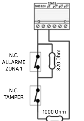
CONTATTO N.C. DI ALLARME E CONTATTO N.C. DI TAMPER CON RESISTENZE DI DOPPIO BILANCIAMENTO
