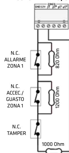
CONTATTO N.C. DI ALLARME ZONA 1, CONTATTO N.C. DI ACCECCAMENTO/ GUAUSTO ZONA 1 E CONTATTO N.C. DI TAMPER CON RESISTENZE DI TRIPLO BILANCIAMENTO
