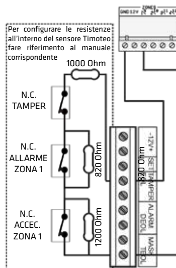
CONTATTO N.C. DI ALLARME ZONA 1, CONTATTO N.C. DI ACCECCAMENTO ZONA 1 E CONTATTO N.C. DI TAMPER CON RESISTENZE DI TRIPLO BILANCIAMENTO ALL'INTERNO DEL SENSORE
