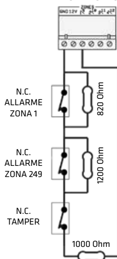
CONTATTO N.C. DI ALLARME ZONA 1, CONTATTO N.C. DI ALLARME ZONA 249 E CONTATTO N.C. DI TAMPER CON RESISTENZE DI TRIPLO BILANCIAMENTO
